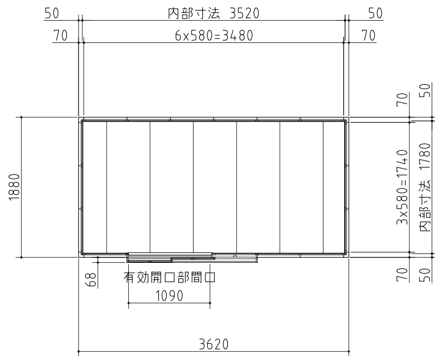
平面図
